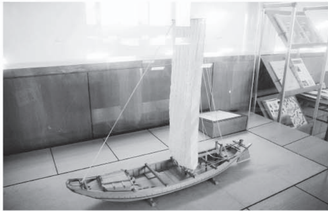
高瀬船
